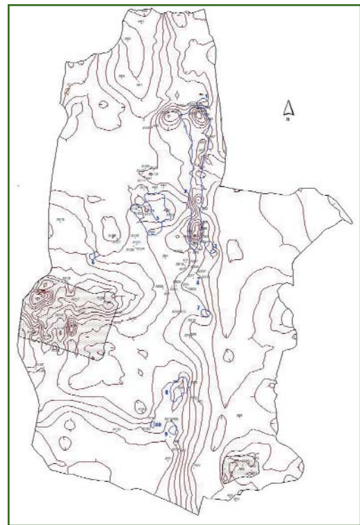
Рис. 6 Топографический план, построенный по результатам GPS-съемки (масштаб 1:4000)
